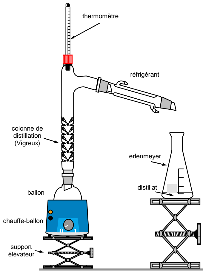
Distillation fractionnée
