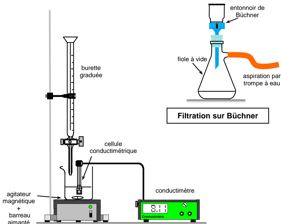
Dosage conductimétrique
